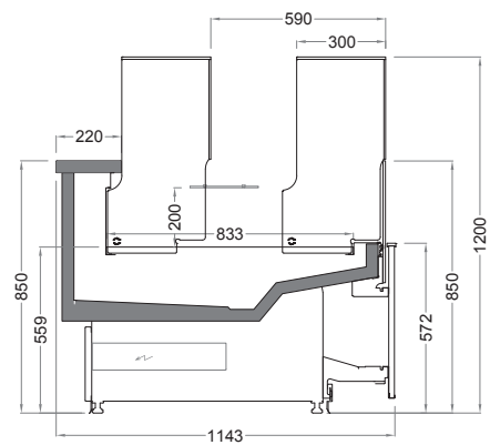
CITRINE CONVERTIBLE 830 / 1200 / 1150 / 540-SQ-D
